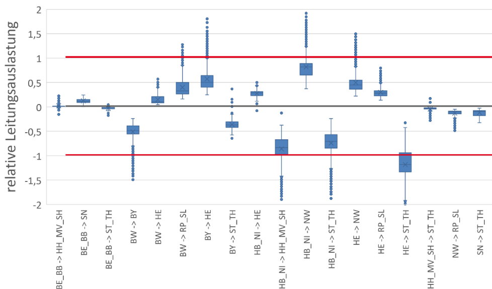
Abb. 8 Austausch zwischen den Regionen
