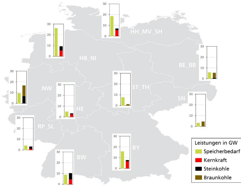
Abb. 7 Vergleich Speicherbedarf - Kernkraftwerksanschlussleistung Fraunhofer ISE
