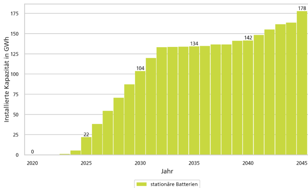
Abb. 3 Entwicklung stationäre Batteriespeicher (Szenario »Referenz«) Fraunhofer ISE
